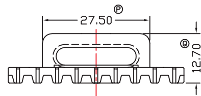
A向视图
