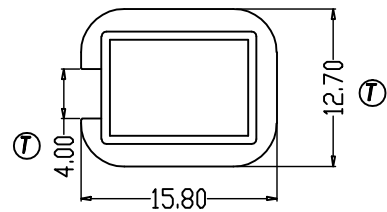
A-A截面图
