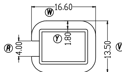
A-A截面图
