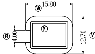
A-A截面图
